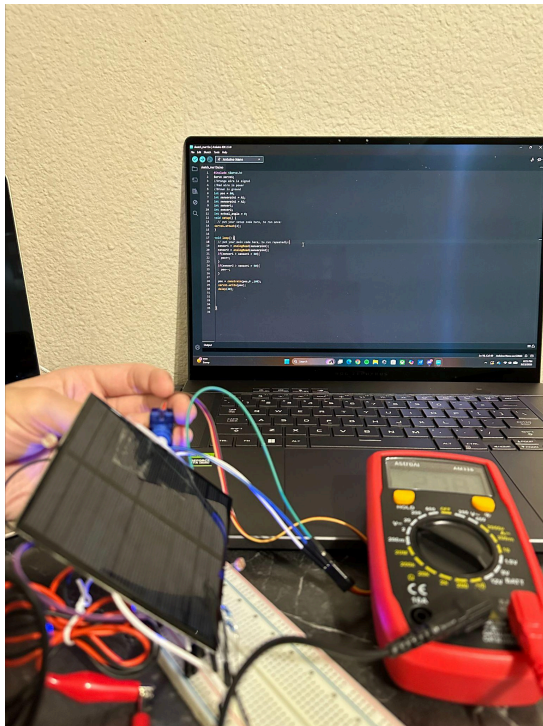
Arduino solar tracker:
